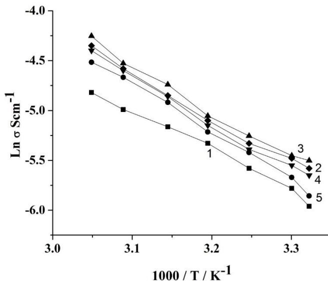
Figure 1 : Temperature dependence of conductivity of PVdF / 1B3MITF / ZnTF GPE with the salt concentration (1- IL : Polymer = 2 : 1, 2 - IL : Polymer : salt = 2 : 1 : 2, 3 - IL : Polymer : salt = 2 : 1 : 2.5, 4 - IL : Polymer : salt = 2 : 1 : 3, 5 - IL : Polymer : salt = 2 : 1 : 5)
