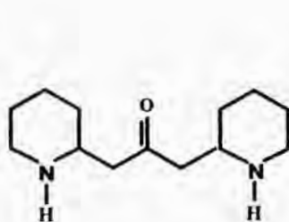
Anaferine
