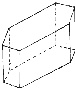
MONOCLINIC
