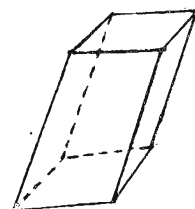
TRICLINIC
