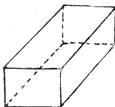
ORTHORHOMBIC
